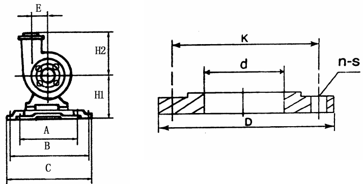
B、泵进出口法兰间图
